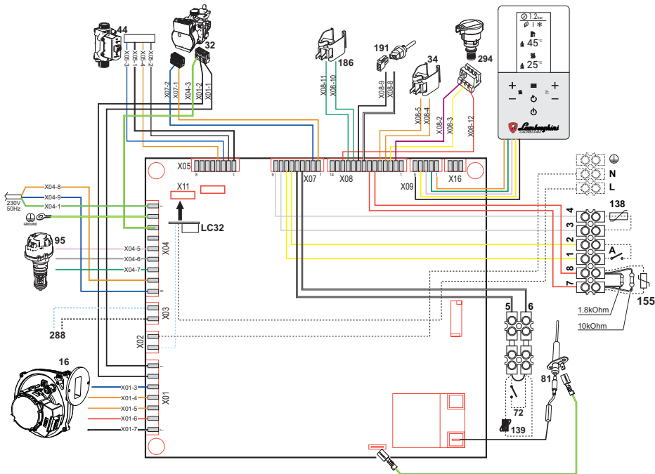
fig. 66 - Schema elettrico
