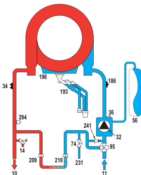
fig. 62 - Circuito idraulico
