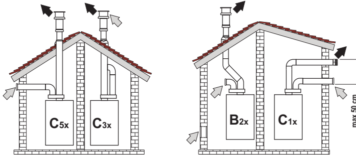
fig. 33- Ejemplos de conexión con tubos separados (⇨ = aire / ⇨ = humos)
