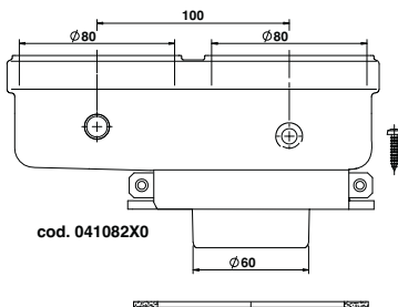
wygląd 34- Człon początkowy do montażu oddzielnych przewodów
