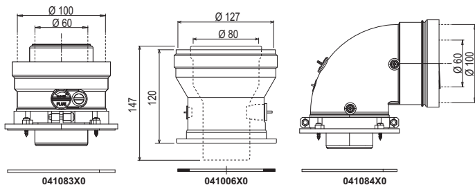
εικ. 32- Εξαρτήματα σύνδεσης για ομοαξονικούς αγωγούς
