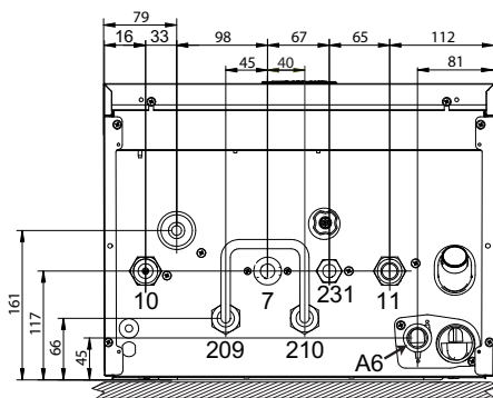
fig. 60- Vista inferior
