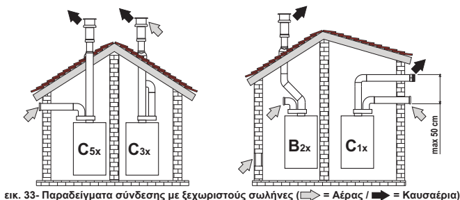
εικ. 33- Παραδείγματα σύνδεσης με ξεχωριστούς σωλήνες (A = Αέρας / B = Καυσαέριο)
