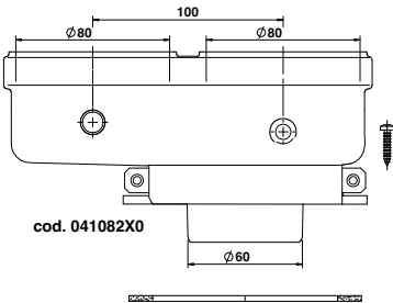
fig. 34 - Accessorio di partenza per condotti separati
