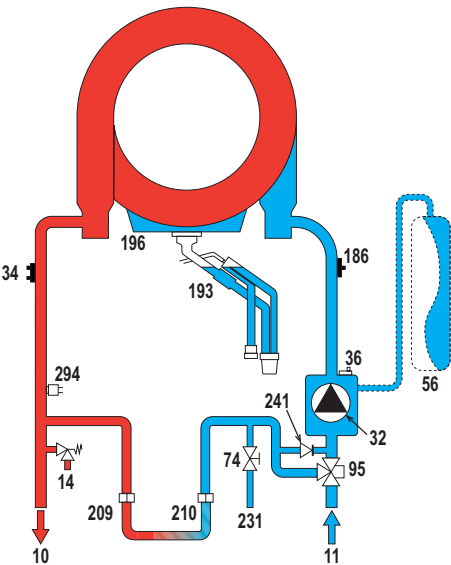
fig. 62- Circuito hidráulico
