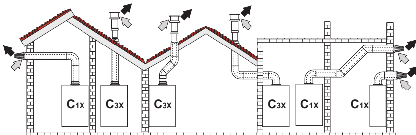
wygląd 31- Przykłady połączenia przewodami współosiowymi (⇨ = Powietrze / ⇨ = Spaliny)
